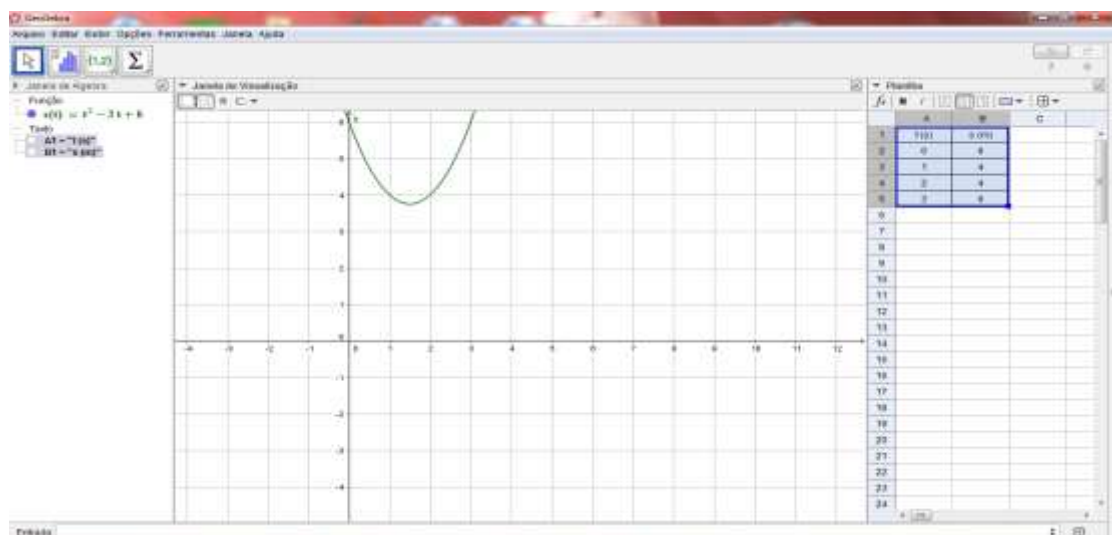
Figura 8: Gráfico da posição em função do tempo [ s = f(t) ] para a função horária s = 6 - 3.t + t^2 (SI).
